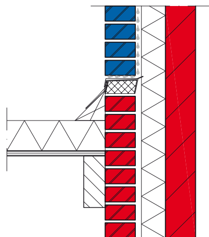
Detail aansluiting plat dak tegen bestaand metselwerk met Ubbink Isolatiesteen
