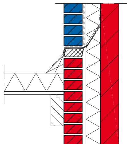
Detail nieuwbouw met Ubbink spouwprofiel i.v.m. valspectie
