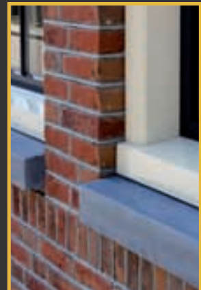
VERLENGDE ONDERDORPEL
