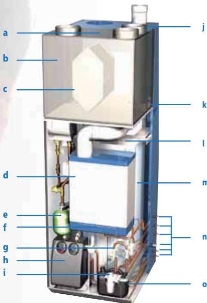
Opengewerkt Passiefhuistoestel
